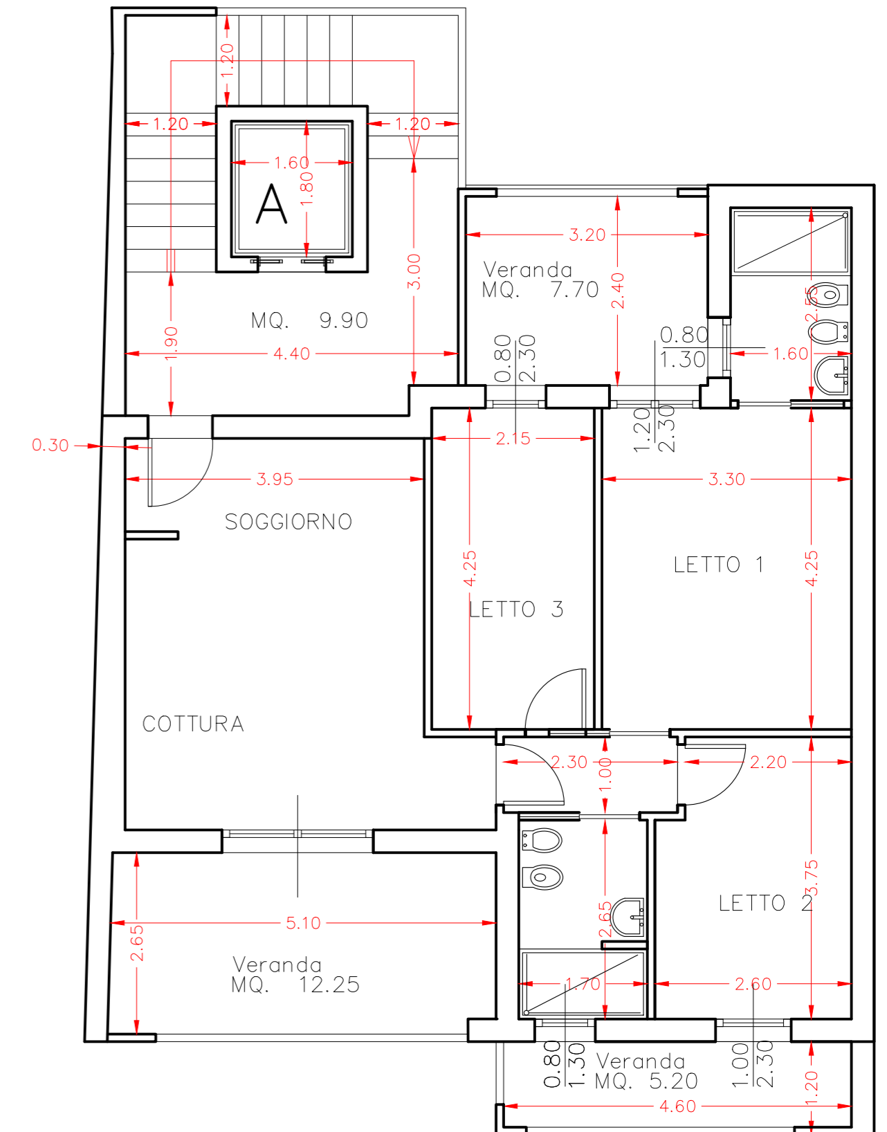
PIANTA P. 3° QUADRIVANO ANGOLO COTTURA
