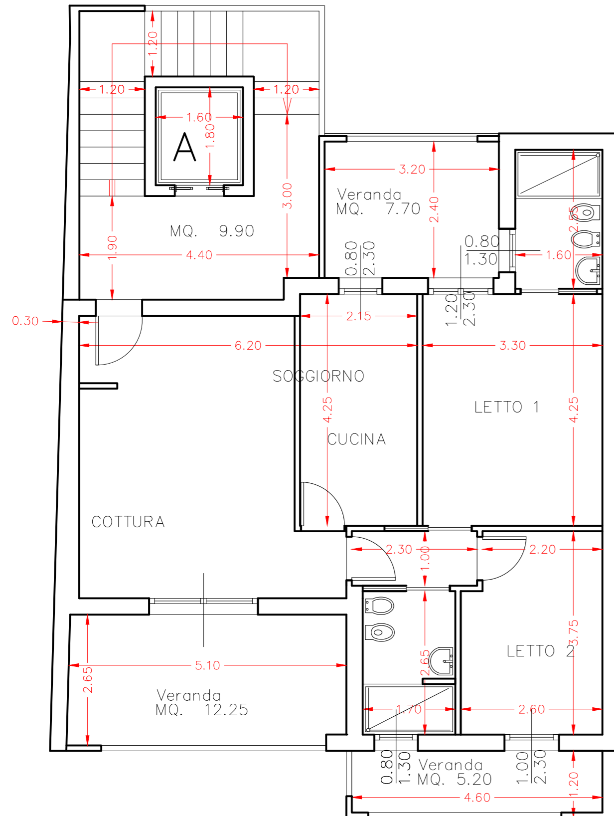
PIANTA P. 3° TRIVANO CUCINA ABITABILE
