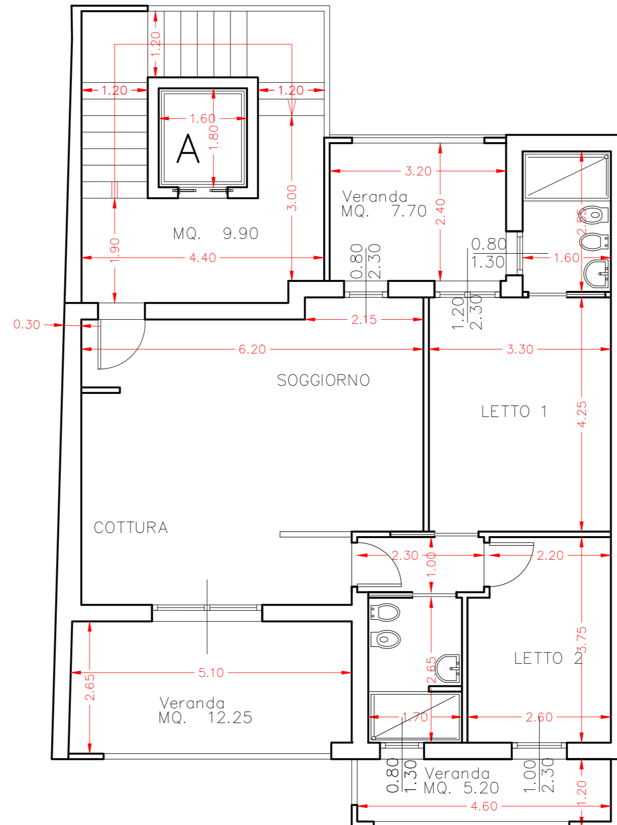
PIANTA P. 3° TRIVANO OPEN SPACE
